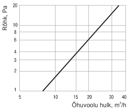
Rõhukao graafik
