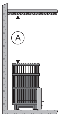
Рисунок 9. Безопасные расстояния (все размеры приведены в миллиметрах)
