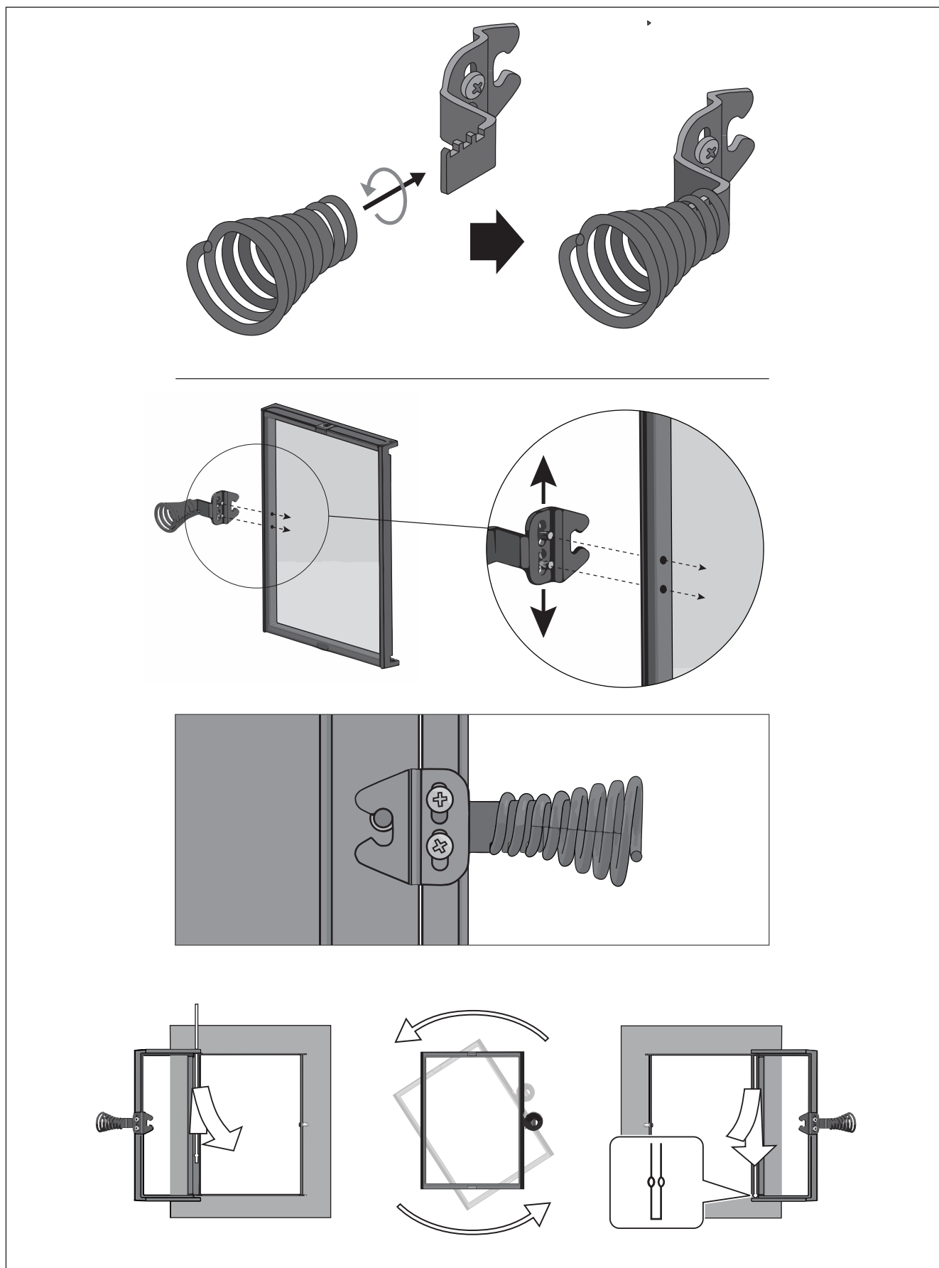
Kuva 13. Luukun käsisyyden vaihtaminen Bild 13. Byte av luckans öppningsriktning
