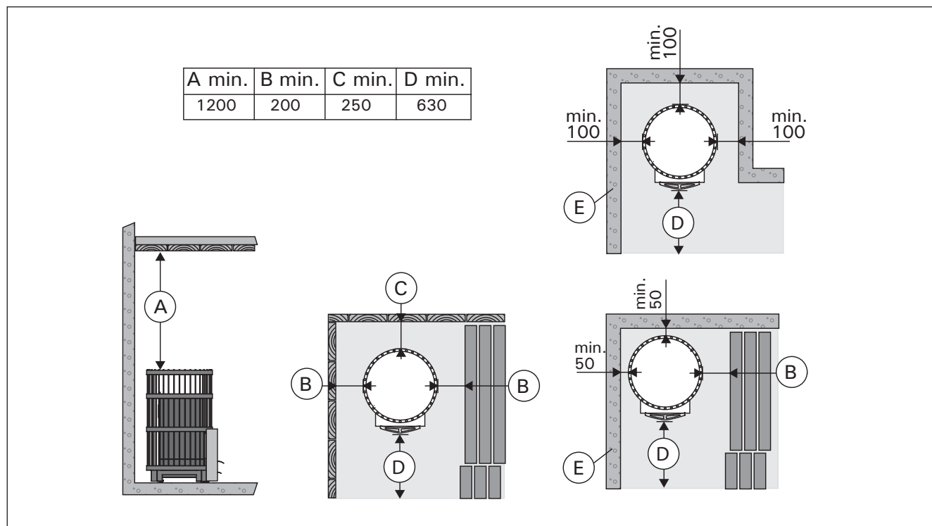
Kuva 9. Suojaetäisyydet (mitat millimetreinä) Bild 9. Säkerhetsavstånd (mått i millimeter)
