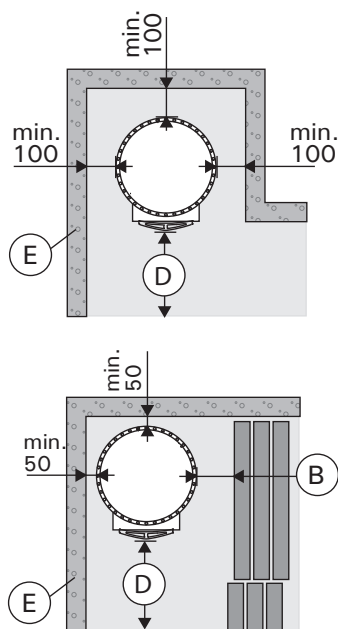
Рисунок 9. Безопасные расстояния (все размеры приведены в миллиметрах)
