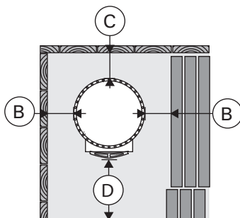
Рисунок 9. Безопасные расстояния (все размеры приведены в миллиметрах)
