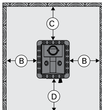
7. zīm. Droši attālumi (visi izmēri norādīti milimetros) 7 pav. Saugūs atstumai (visi matmenys - milimetrais)
